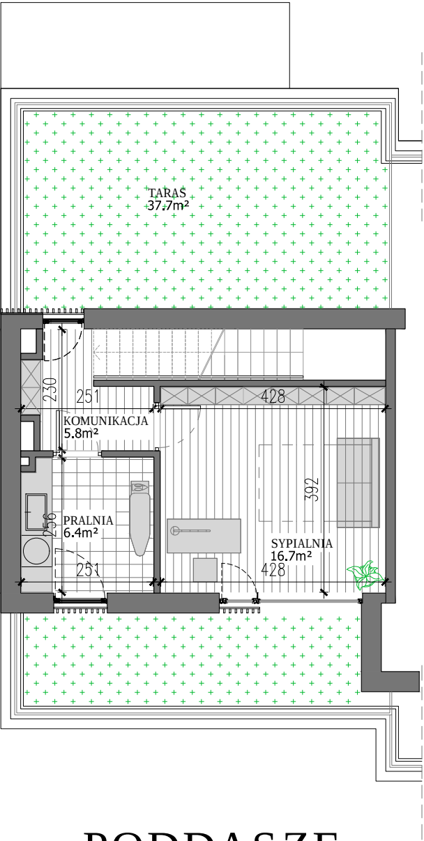
PODDASZE
